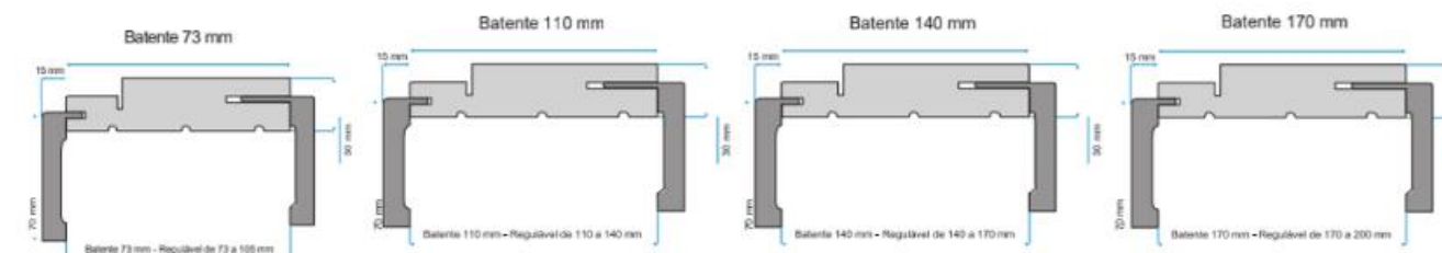
K73-701 Kit Batente-Guarnição Regulável 73 a 105 mm
